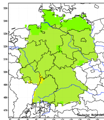
WETTREG
