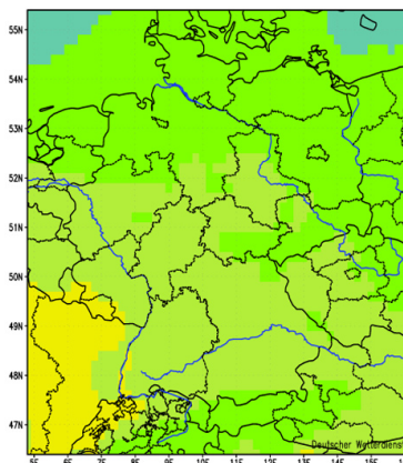
CLM
