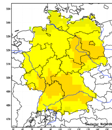
STAR
